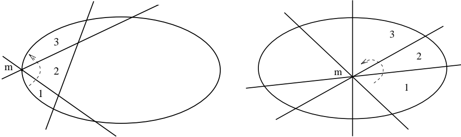
Fig. 2.5. m = m(\Omega) or m \in \text{int } \Omega .
