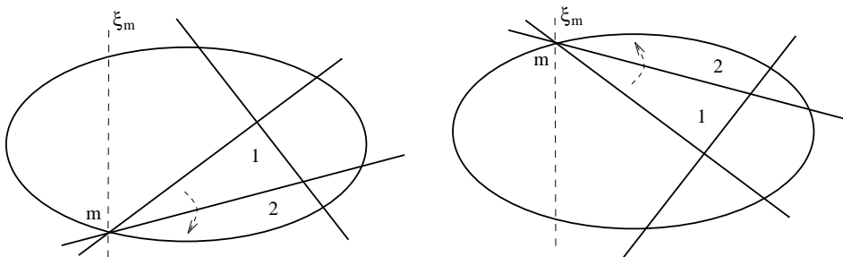
Fig. 2.6. m \in \partial\Omega \setminus \{m(\Omega)\} .
